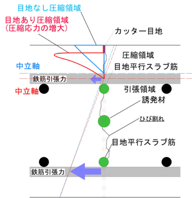
図2 曲げ抵抗機構
