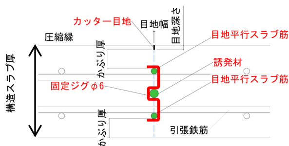
図1 目地部構成部材
