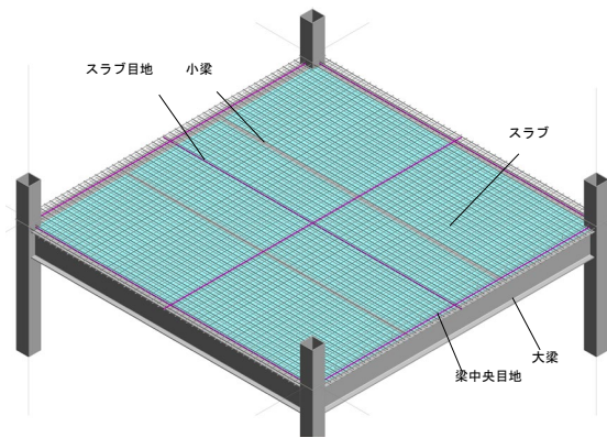
図3 目地位置 (S造架構例)
